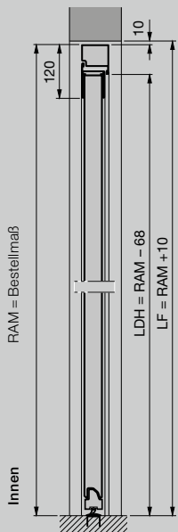
Nebentür mit Alu-Blockzarge Profiltyp 2 Einbau in der Öffnung
