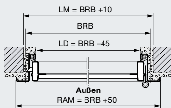
Außenanschlag nach außen öffnend
