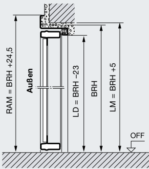
Außenanschlag nach außen öffnend
